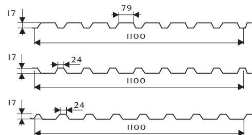
Trapézlemez T20
