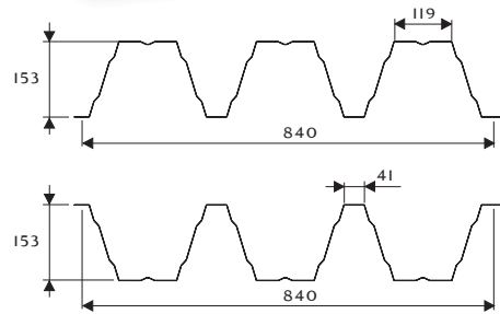
Teherhordó T153
