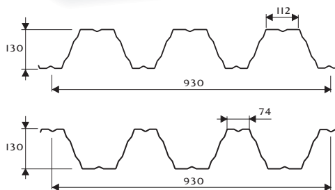
Teherhordó T130
