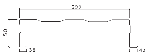
C-zazetta LT150
